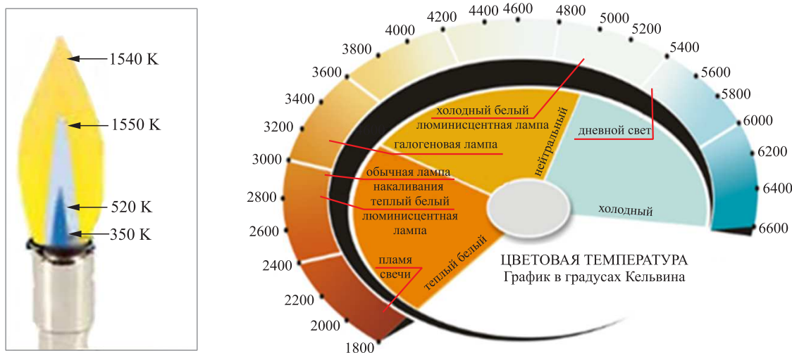
Рис. 3 Цветовая температура в источниках света
