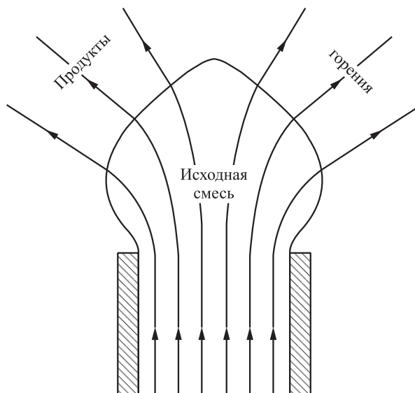
Рис. 2 Линии тока газовой смеси вблизи среза горелки
